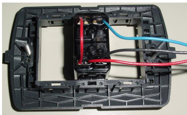
Pulsanti collegati
