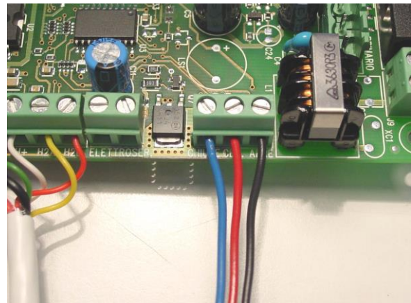
Collegamento dei conduttori dei pulsanti alla centralina.
