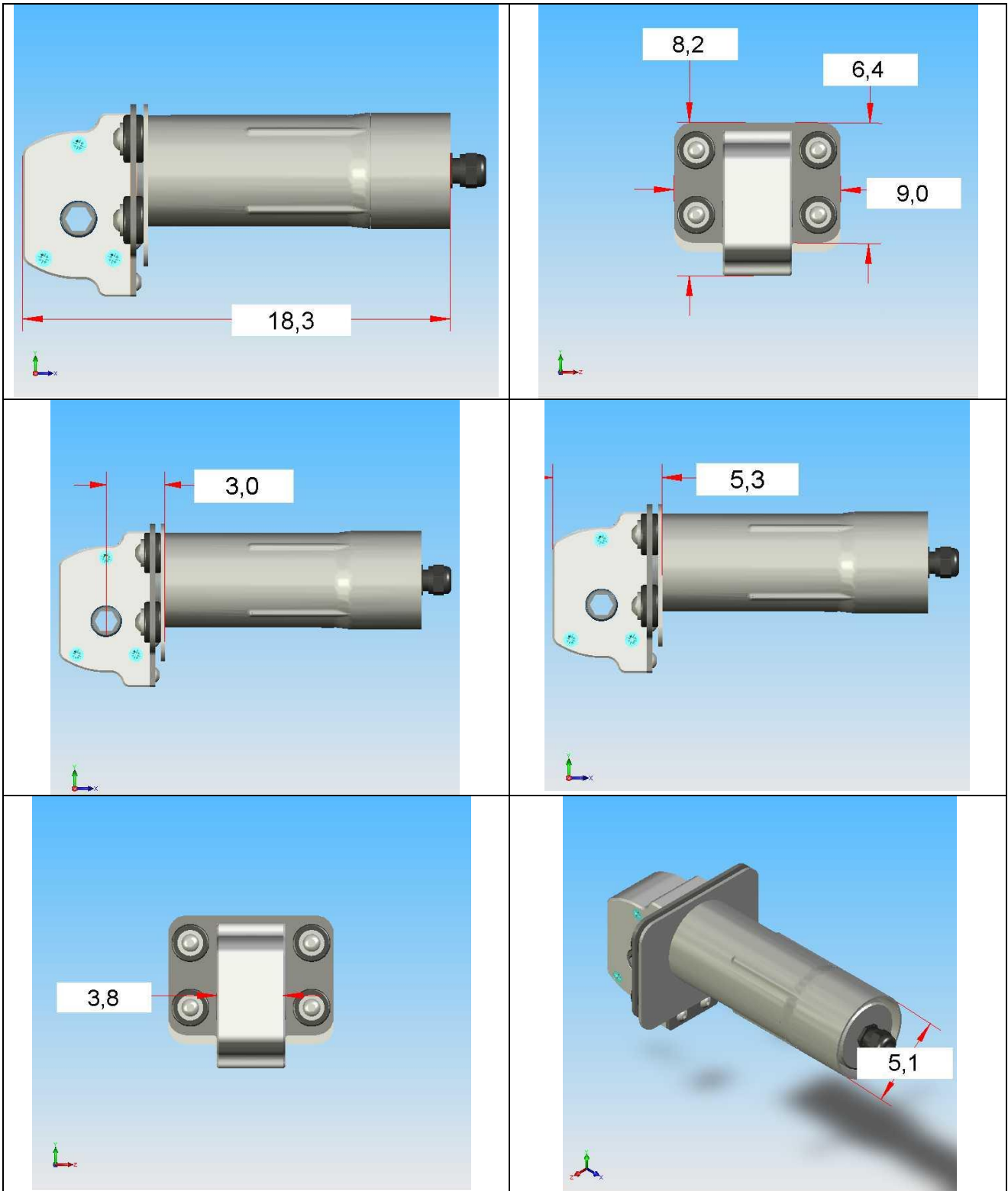
Misure del motoriduttore Click! Slim (in centimetri)
